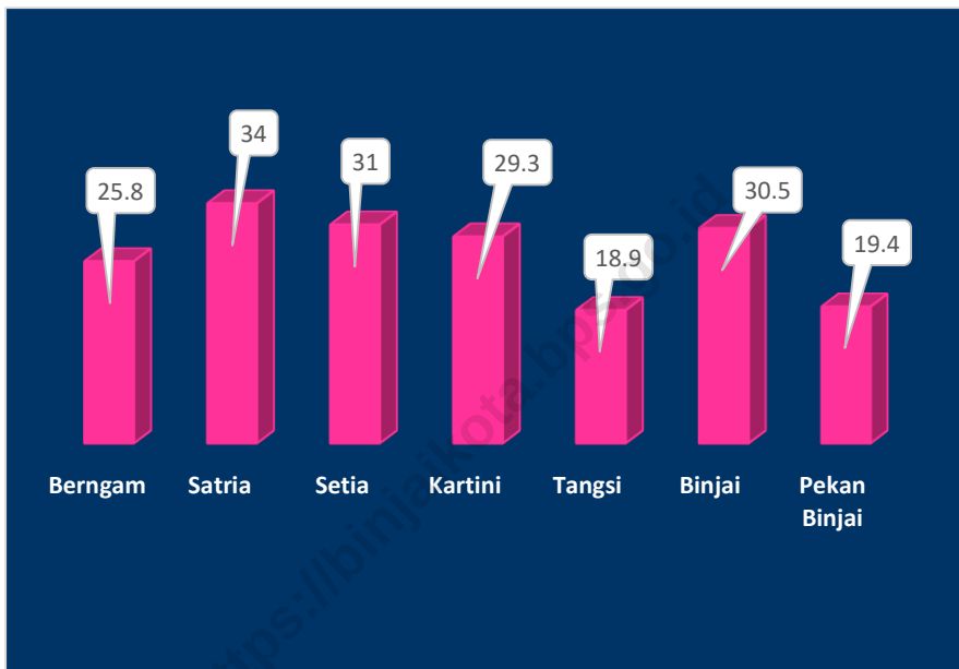
Gambar 1.2 Tinggi Wilayah di Atas Permukaan Laut (DPL) Menurut Kelurahan di Kecamatan Binjai Kota, 2019 Height Above Mean Sea Level (AMSL) of Binjai Kota Sub district by Locality , 2019
