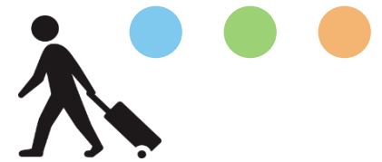
Jumlah Penumpang
