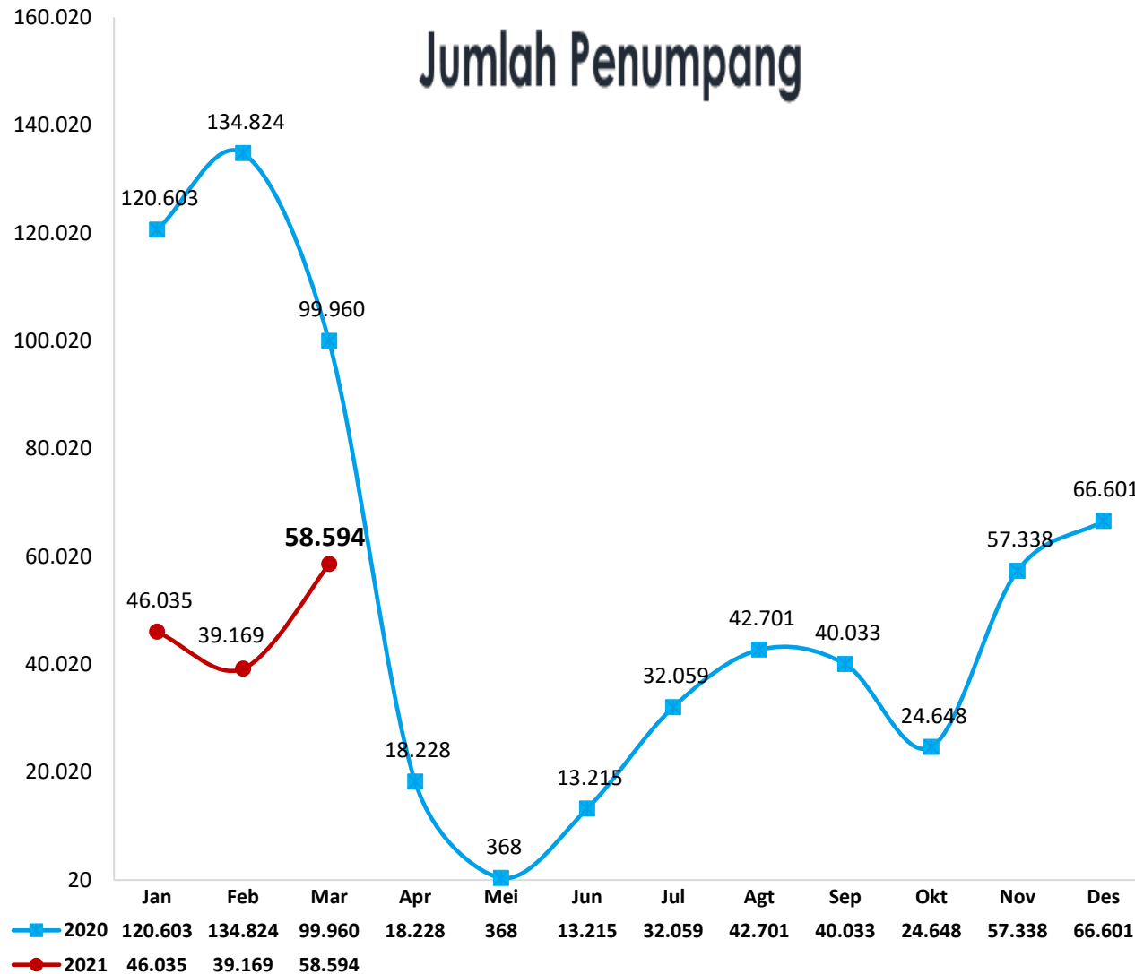
Jumlah Penumpang
