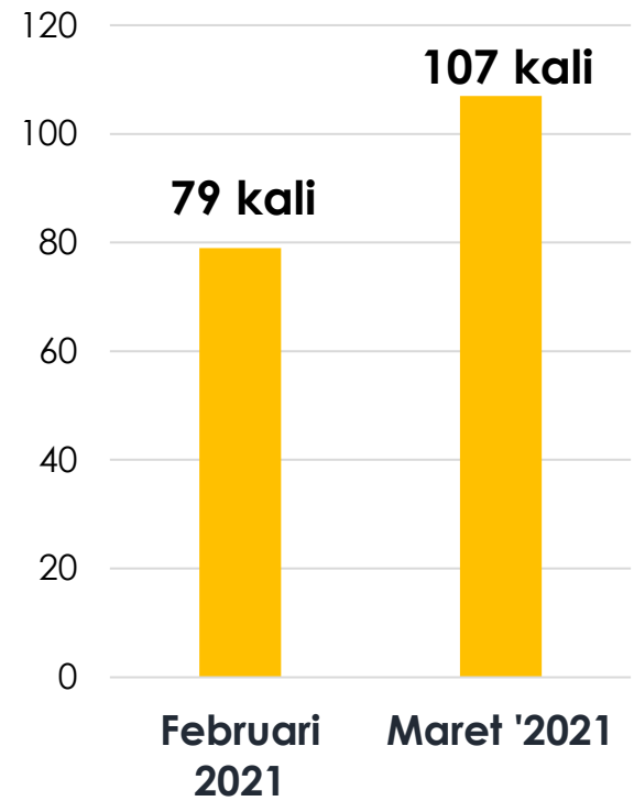
Frekuensi Pelayaran
