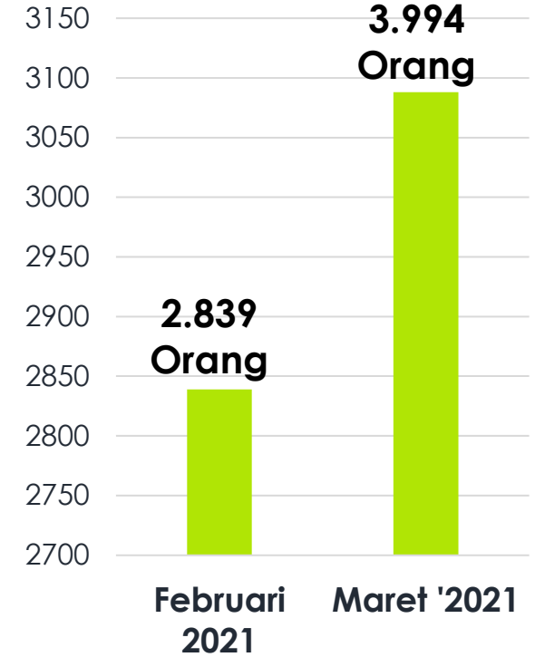
Jumlah Penumpang
