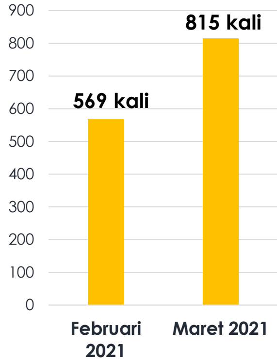
Frekuensi Penerbangan
