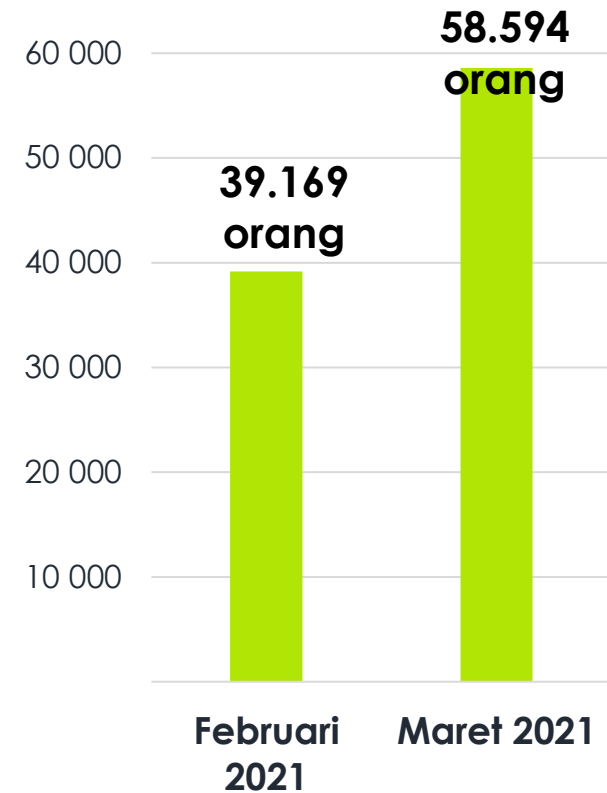
Jumlah Penumpang
