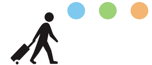
Jumlah Penumpang
