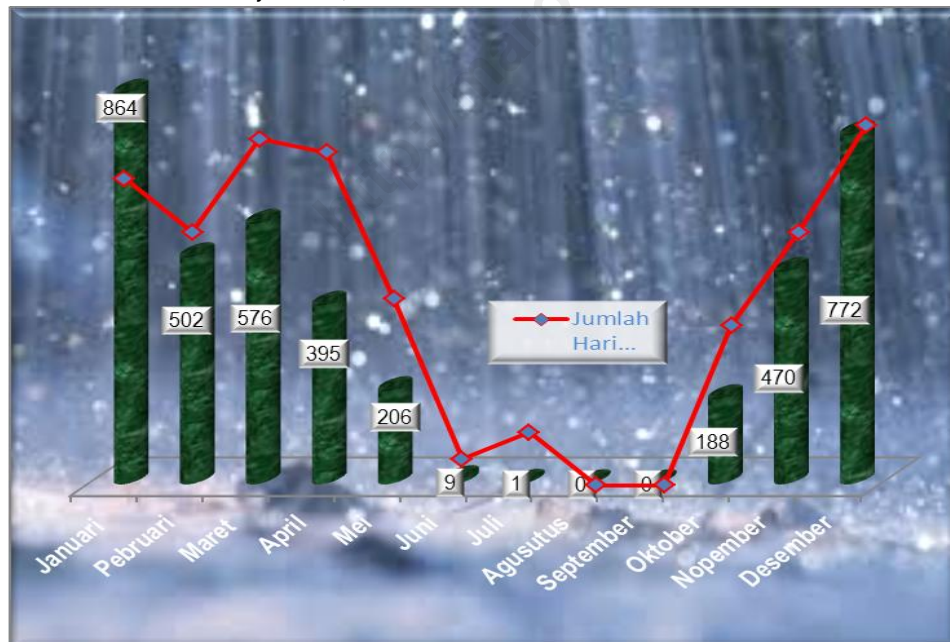
Grafik 1.2 Jumlah Curah Hujan dan Banyaknya Hari Hujan Menurut Bulan Tahun 2011 di Maros
