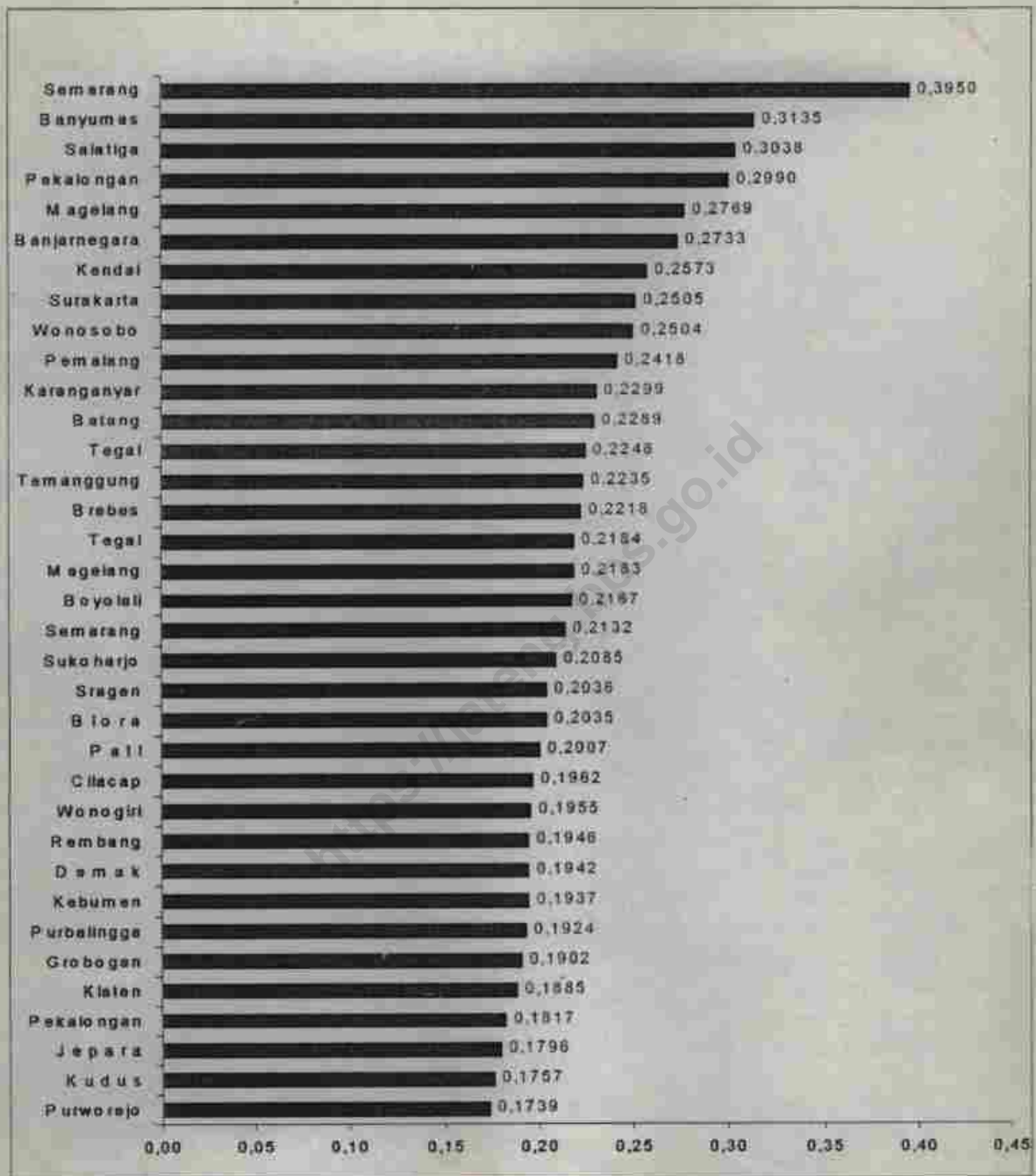
Gambar 2 Nilai Gini Rasio Yang Sudah Diurutkan
