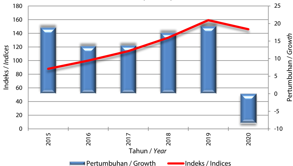
Gambar/Figure 15.6. Benchmark Indeks dan Pertumbuhan Nilai Konstruksi yang Diselesaikan Provinsi Jawa Timur (2016=100) Benchmarked Indices and Benchmarked Growth of Value of Construction Completed of Jawa Timur (2016=100)
