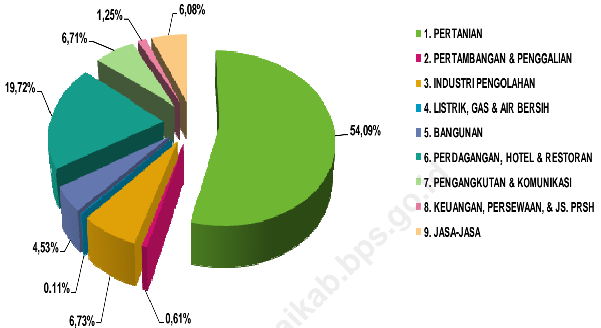
GRAFIK 3.2 DISTRIBUSI PERSENTASE PDRB KABUPATEN KEPULAUAN MENTAWAI/ DISTRIBUTION GRDP OF KEPULAUAN MENTAWAI REGENCY 2011
