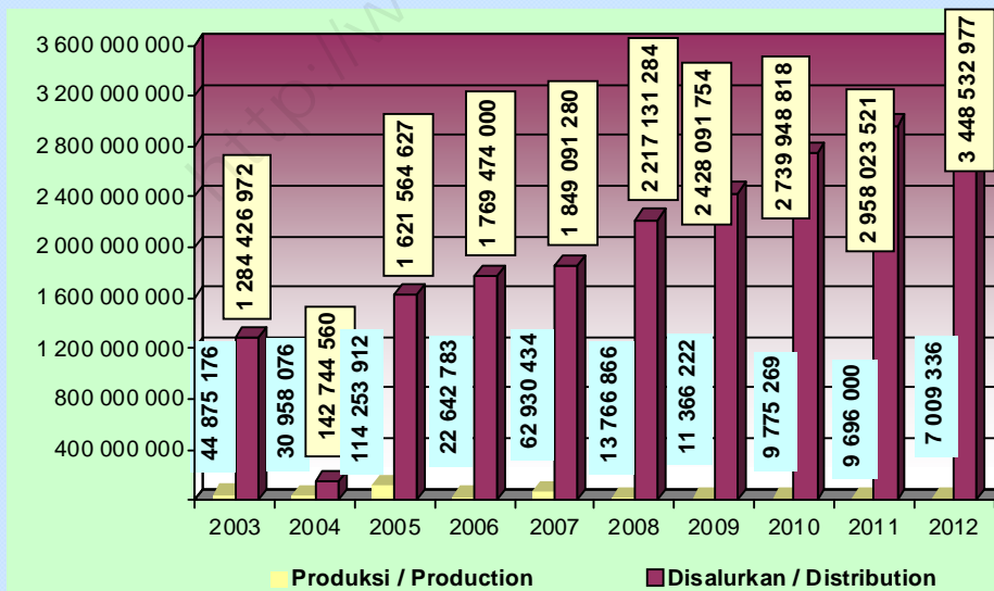
Gambar 6.2. Jumlah Tenaga Listrik yang Diproduksi dan Disalurkan PLN di Sumatera Selatan (KWh), 2003-2012 Figure Electricity Produced and Distributed by PLN in Sumatera Selatan (KWh), 2003-2012
