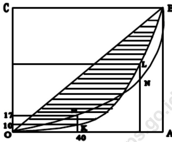
Gambar 1. Kurva Lorenz
