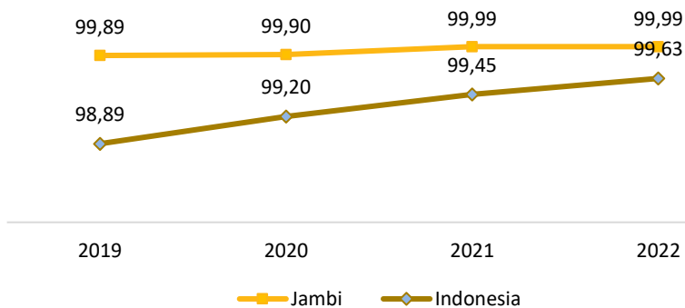
GAMBAR 7.1 RASIO ELEKTRIFIKASI DI PROVINSI JAMBI DAN INDONESIA (PERSEN), 2019-2022
