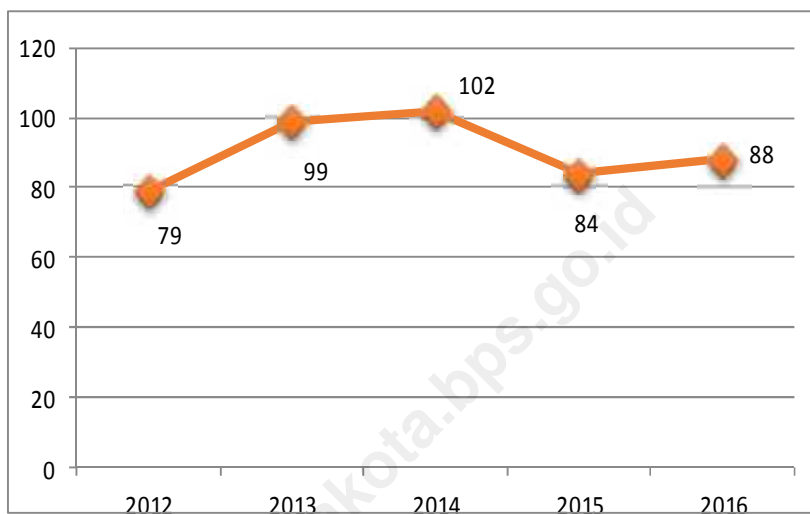
Gambar 1.5 Jumlah Hari Hujan Tahun 2012 - 2016 (hari) Number of Rainydays, 2012 - 2016 (days)
