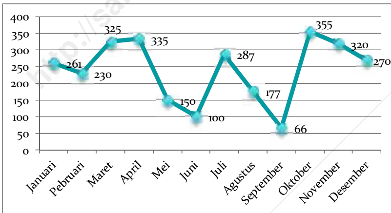
Gambar 1.2 Curah Hujan per Bulan, Tahun 2016 (mm) Rainfall per month, 2016 (mm)
