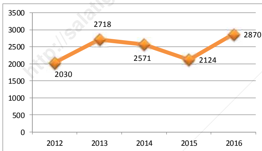
Gambar 1.4 Curah Hujan Tahun 2012 - 2016 (mm) Rainfall 2012 - 2016 (mm)
