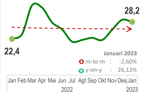
Nikel (000 $/mt)
