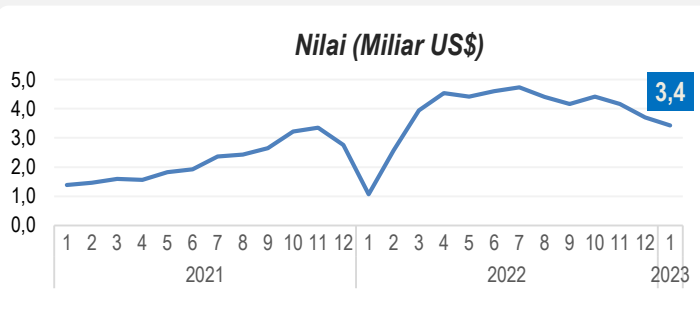
Batu Bara
