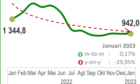
Nikel (000 $/mt)
