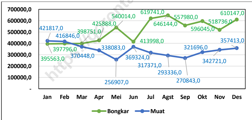
Gambar 18. Jumlah Bongkar Muat Barang (Kargo, Bagasi, dan Pos/Paket) Melalui Bandara Jalaluddin Tahun 2017 (ton)
