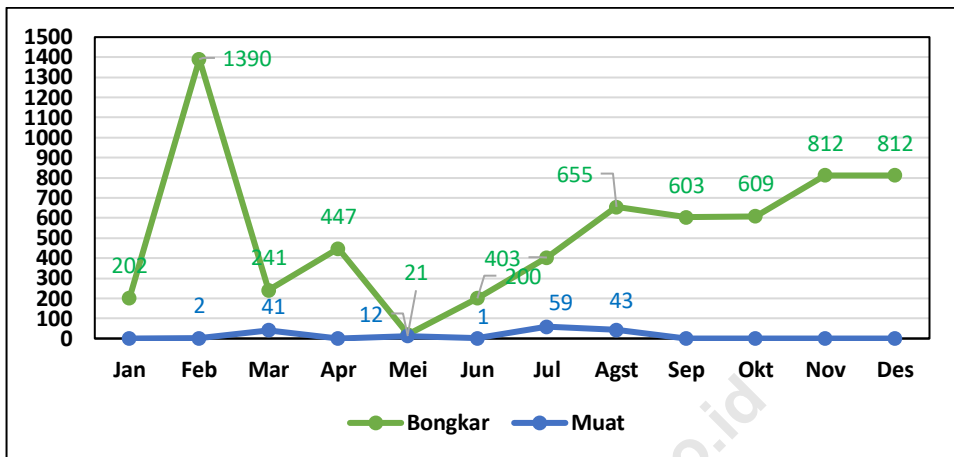
Gambar 6. Jumlah Bongkar Muat Barang di Pelabuhan Kwandang Tahun 2017 (ton)
