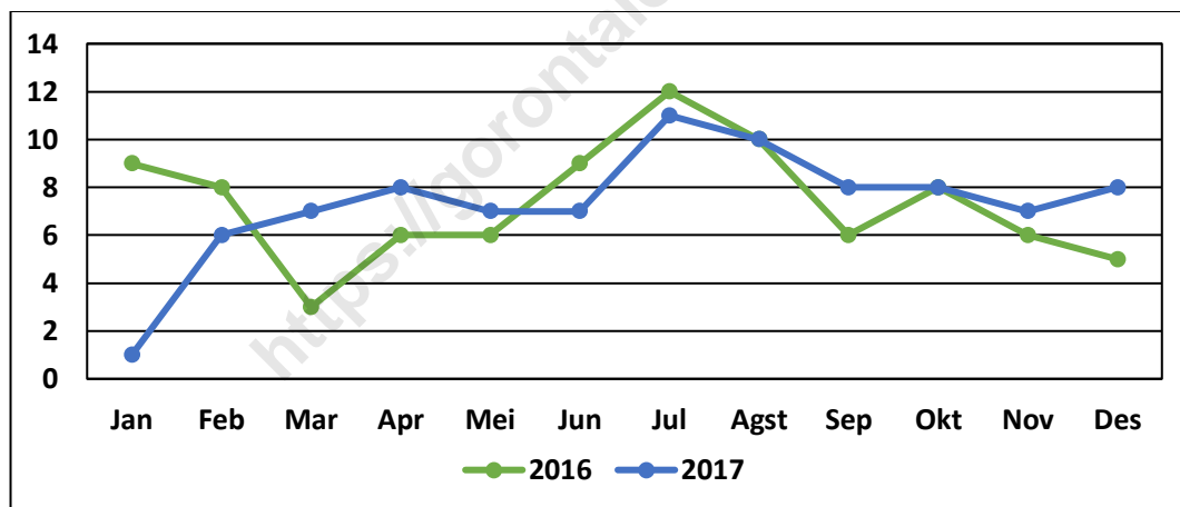
Gambar 4. Jumlah Kapal yang Keluar Masuk Pelabuhan Kwandang Tahun 2016-2017 (unit)
